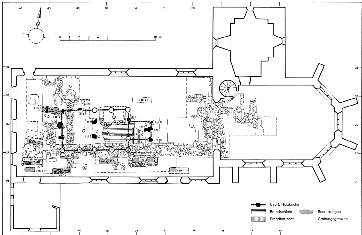
Kornwestheim, St. Martin. Plan der Holzkirche (630/40 bis ca. 750) mit Bestattungen
